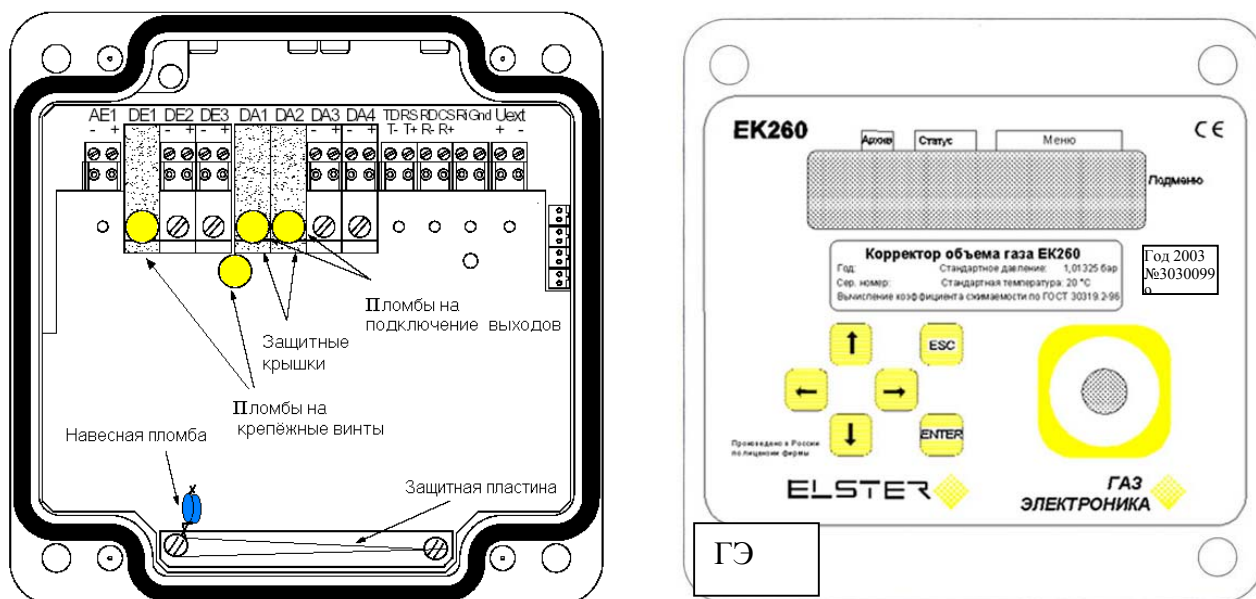
Рис. 2 Расположение пломб
